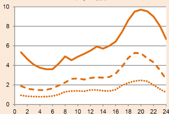
HUSHÅLLSEFFEKT ( \text{W/m}^2_{\text{BOA}} )
