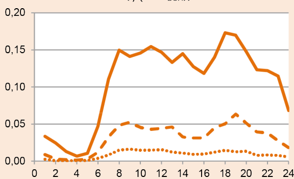
VARMVATTENFLÖDE ( \text{l}/(\text{h} \cdot \text{m}^2_{\text{BOA}}) )
